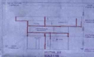
SECTION X-X SCALE: 1:100
