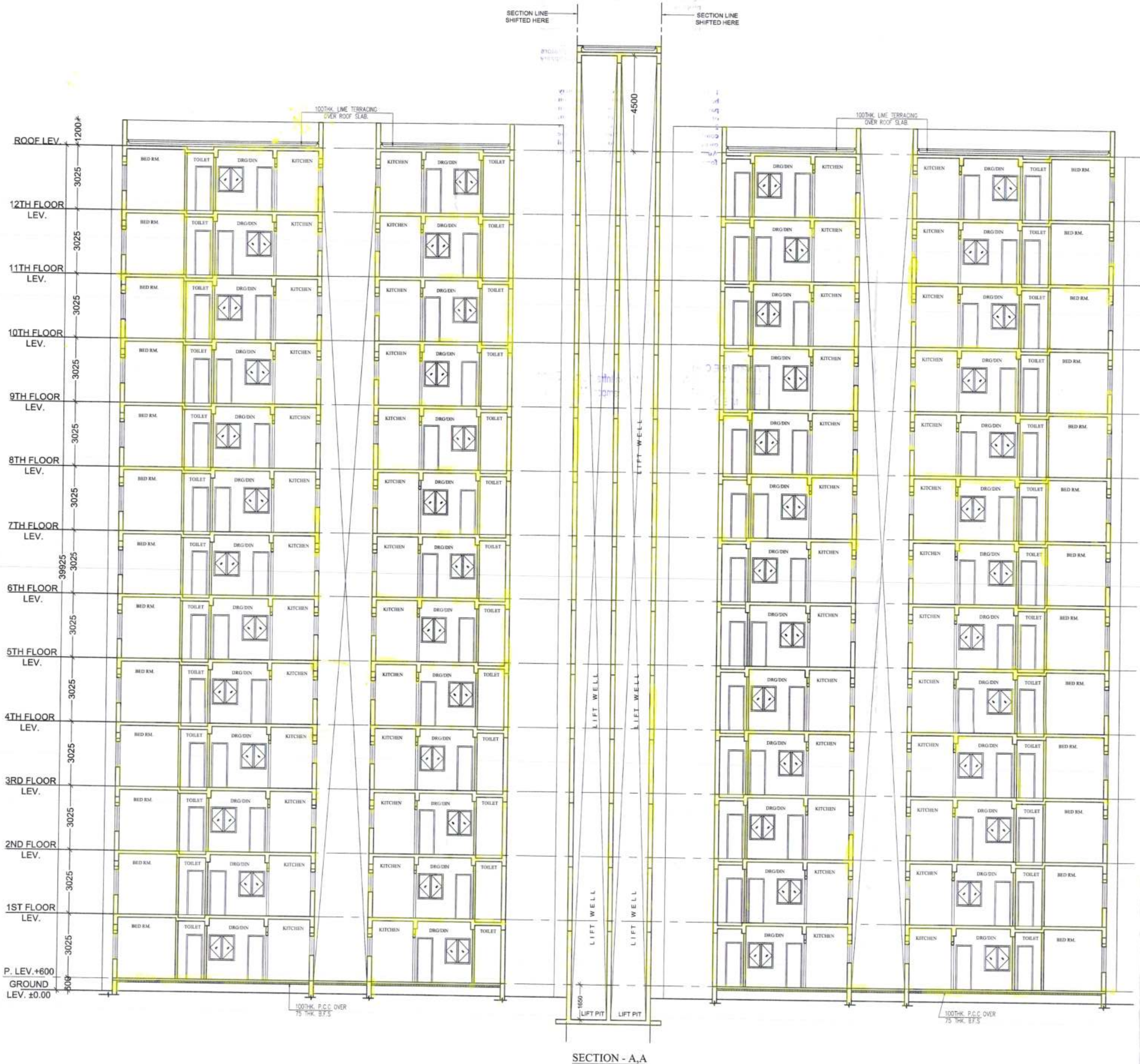
SECTION - A-A
